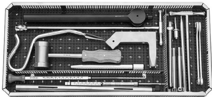
(70140) CAIXA P/ INSTRUMENTAIS P/ HASTE BLOQUEADA FEMORAL UNIVERSAL
