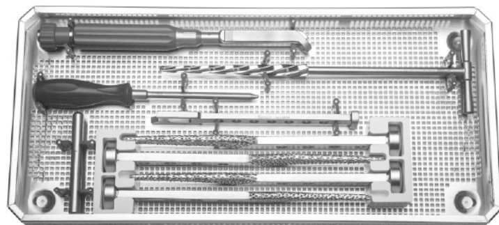
(70241) CAIXA PARA INSTRUMENTAL DE COMPONENTE FEMORAL TIPO MULLER
